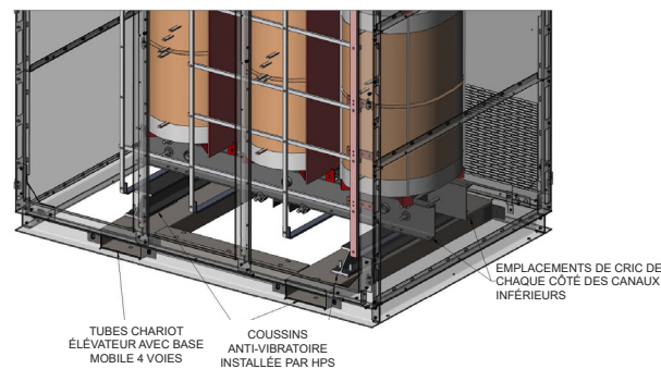
FIGURE 11: BASE OPTIONNELLE POUR CHARIOT-ÉLÉVATEUR AVEC DÉPLACEMENT SUR 4 SENS
