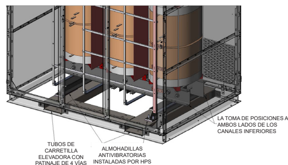
FIGURA 11: OPCIONAL - BASE PARA USO DE MONTACARGAS CON CAPACIDAD DE DESLIZAMIENTO DE 4 VÍAS
